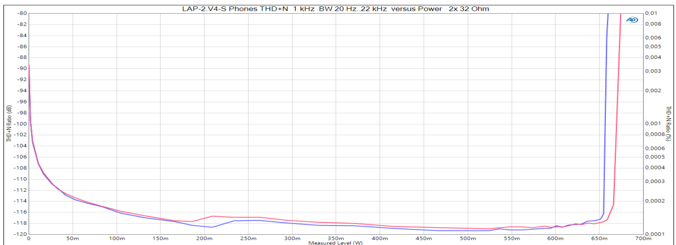
Ausgangsleistung und THD+N-Werte bei 1 kHz und Kopfhörerimpedanz 2x 32 \Omega
