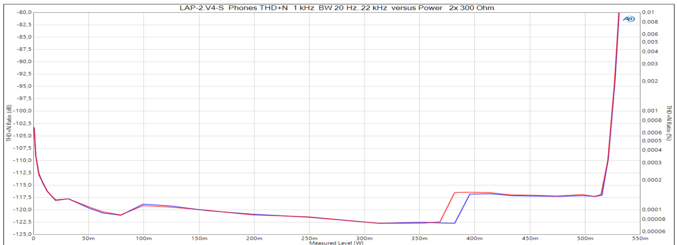
Ausgangsleistung und THD+N-Werte bei 1 kHz und Kopfhörerimpedanz 2x 300 \Omega
