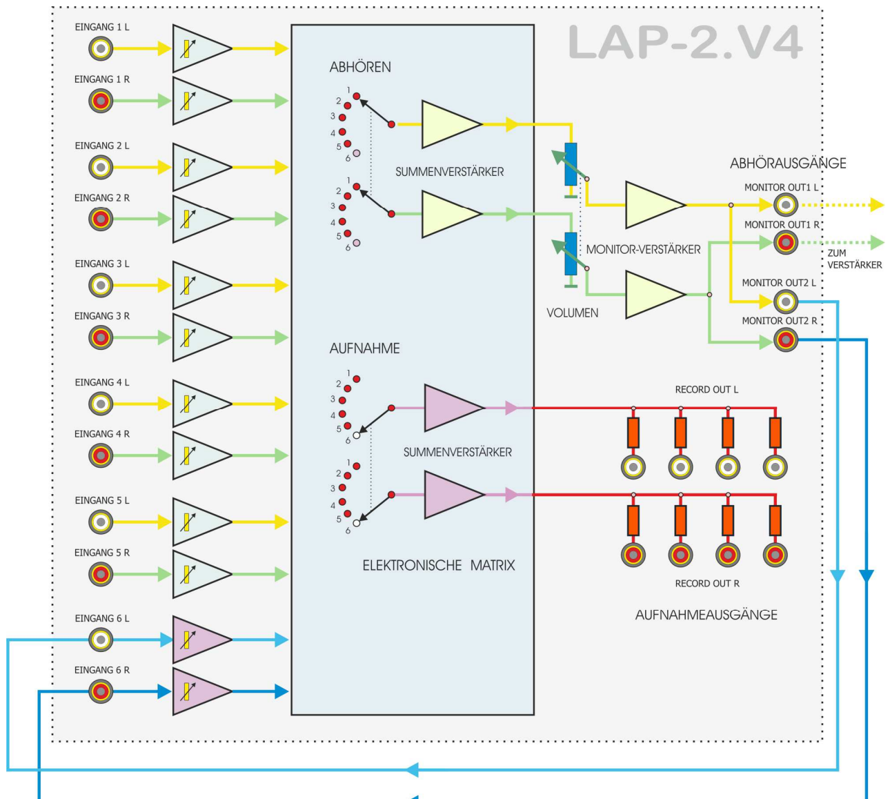
Blockschaltbild ohne Kopfhörerverstärker und Stromversorgung
