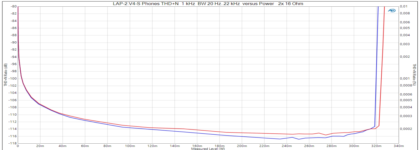
Ausgangsleistung und THD+N-Werte bei 1 kHz und Kopfhörerimpedanz 2x 16 \Omega
