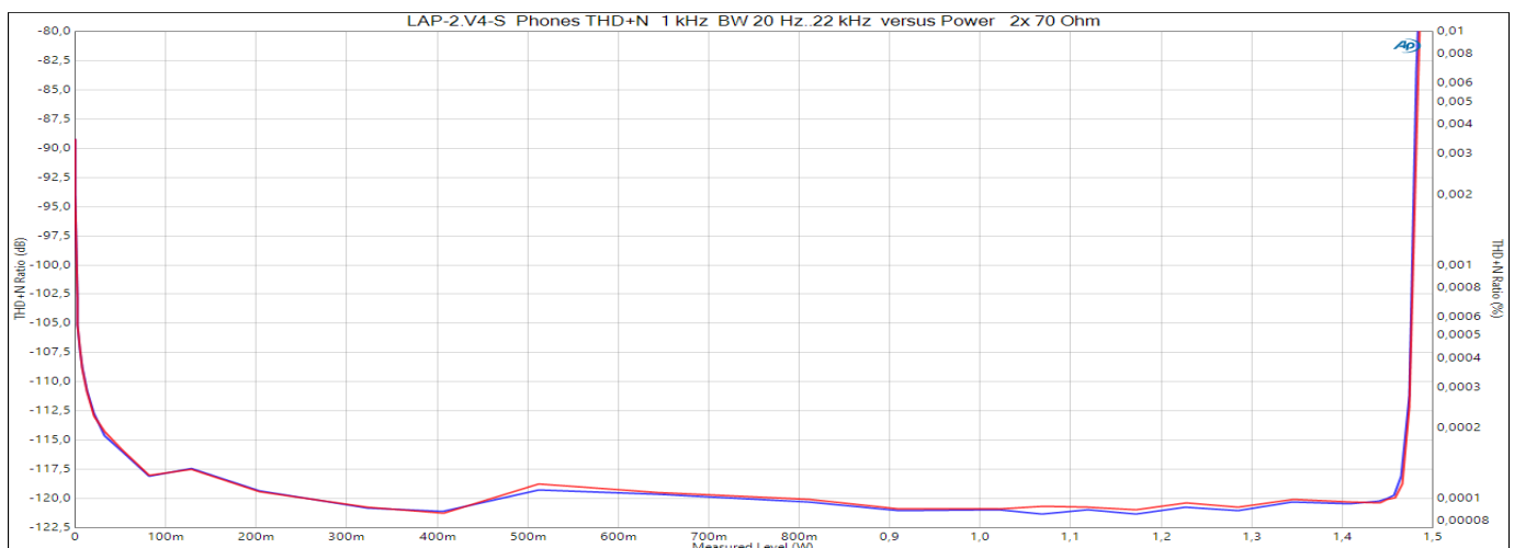
Ausgangsleistung und THD+N-Werte bei 1 kHz und Kopfhörerimpedanz 2x 70 \Omega
