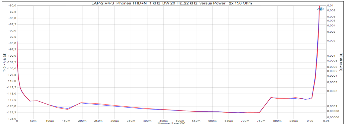
Ausgangsleistung und THD+N-Werte bei 1 kHz und Kopfhörerimpedanz 2x 150 \Omega
