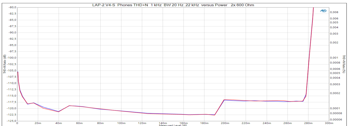
Ausgangsleistung und THD+N-Werte bei 1 kHz und Kopfhörerimpedanz 2x 600 \Omega
