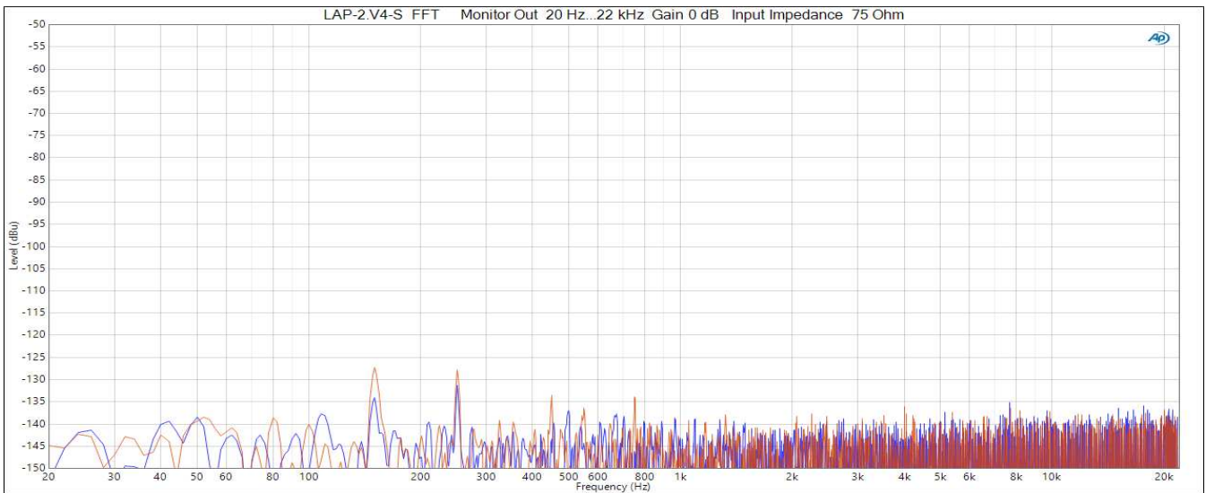
FFT des Rauschens am Ausgang bei Volumenpoti am Rechtsanschlag
